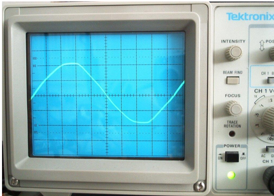
Bild 10 Mit einem Oszilloskop gemessene 50Hz am Tiefpassausgang der Weiche.
